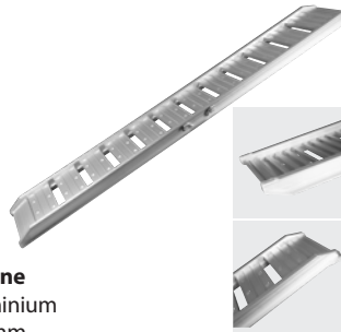
Verladeschiene, klappbar Material Aluminium Bauhöhe 60 mm
